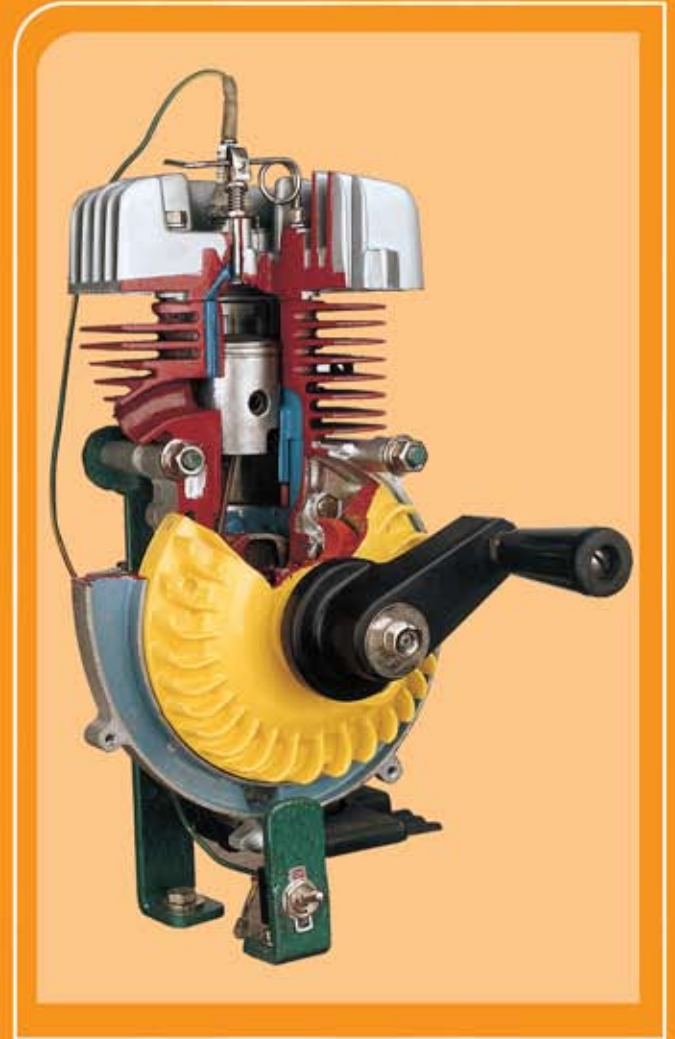
مقطع محرك ثنائي الدورة
